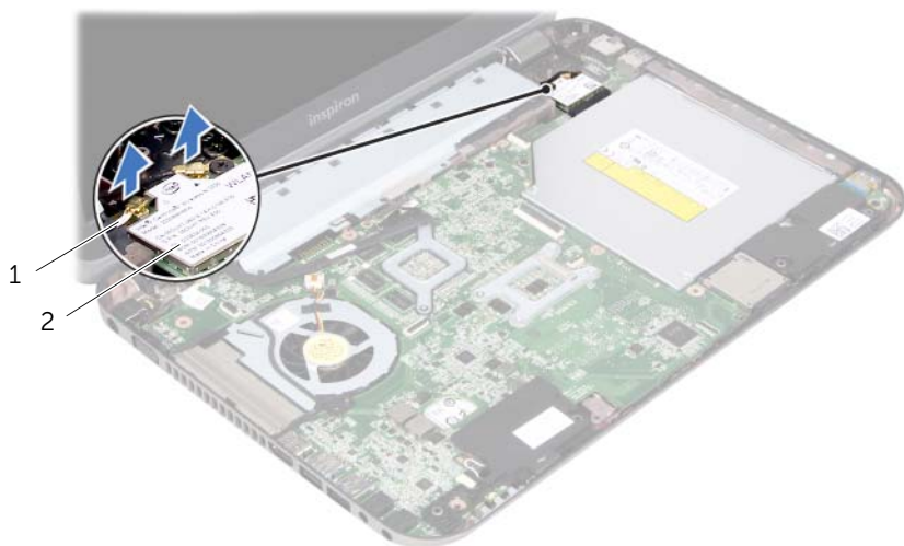
1 antennekabels (2) 2 minikaart
